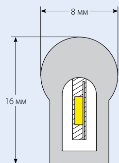
Поперечное сечение светодиодной ленты НЕОН 220 В
